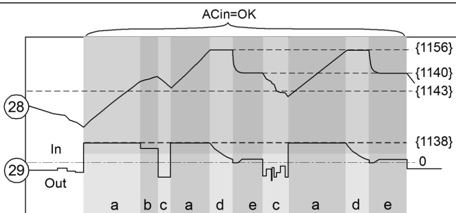
Beispiel eines Batterieladezyklus mit Eingangsstrombegrenzung und Smart-Boost-Funktion
