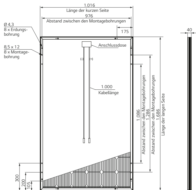
Rahmenquerschnitt
