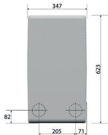
Frontansicht
